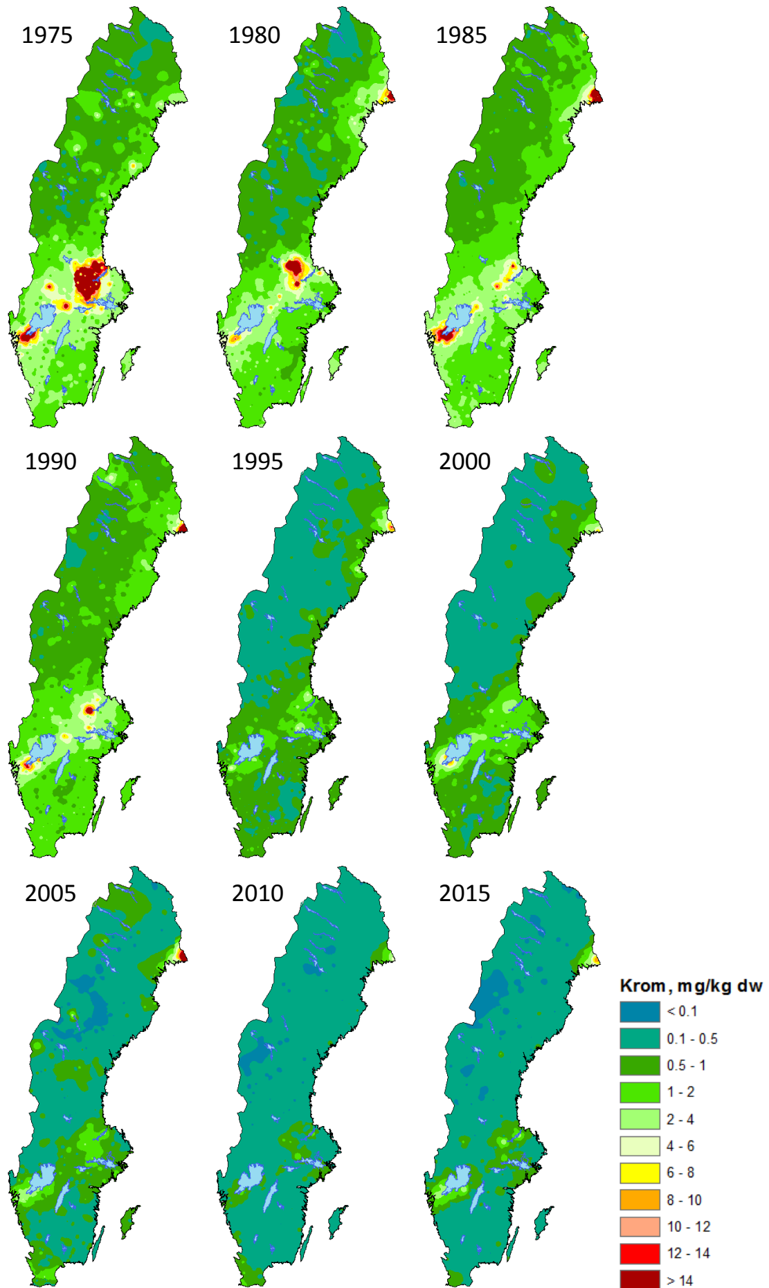
Figur 28. Koncentration (mg/kg torrsvikt) av krom i mossor, 1975-2015.
