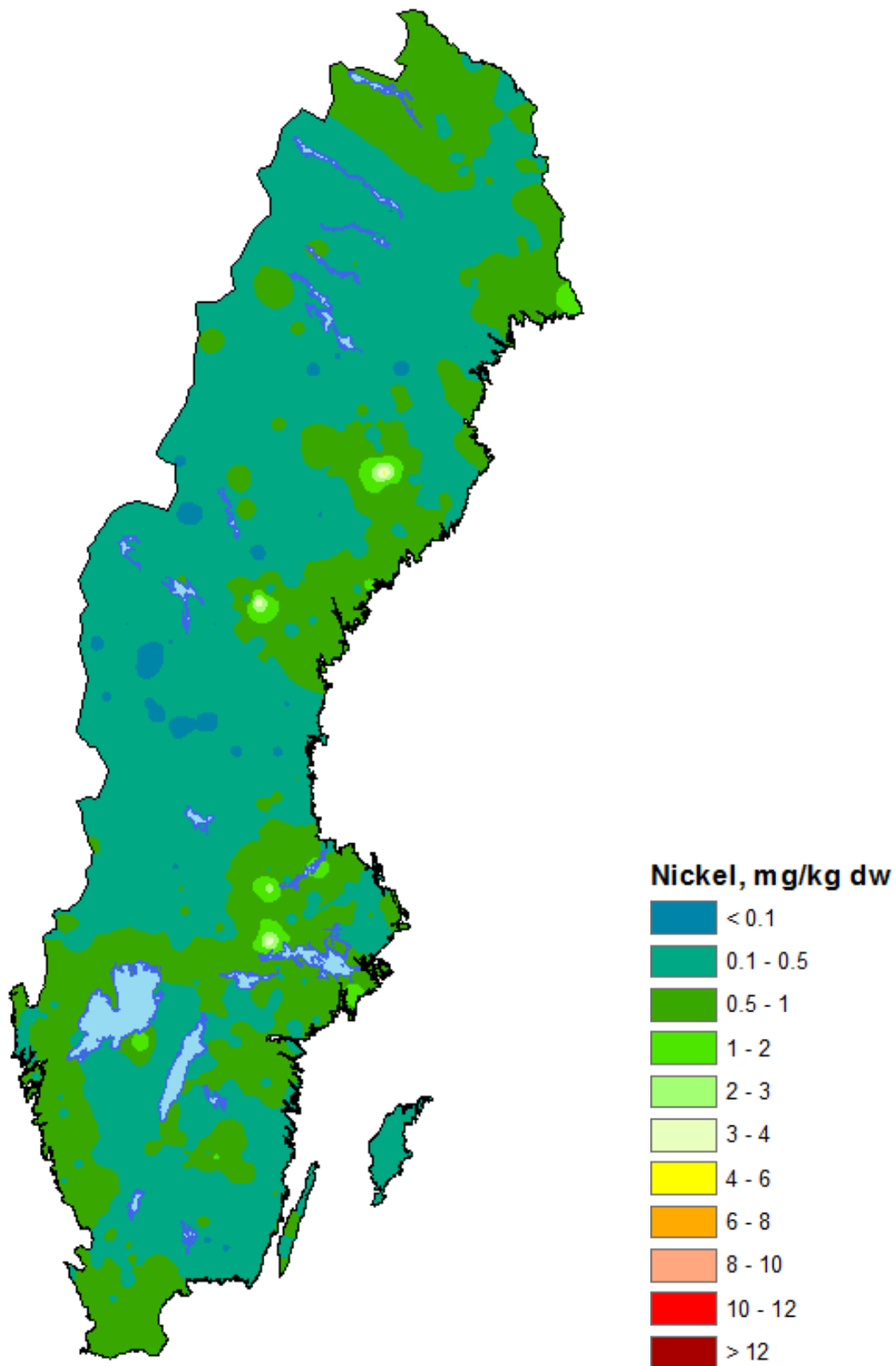
Figur 35. Nickelkoncentrationer i mossprover insamlade 2015.
