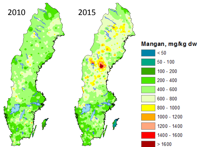
Figur 57. Koncentration (mg/kg torrsvikt) av mangan i mossa, 2010 och 2015.
