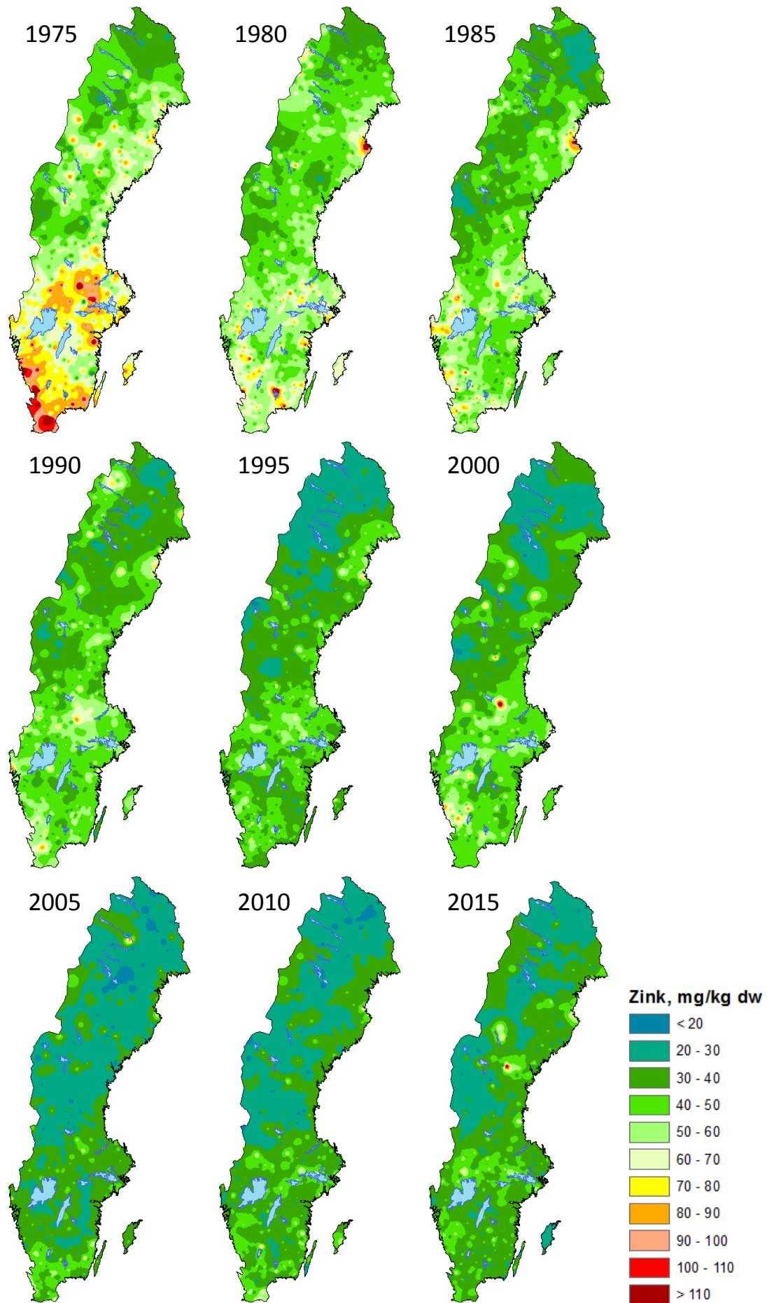
Figur 46. Koncentration (mg/kg torrsvikt) av zink i mossa, 1975-2015.
