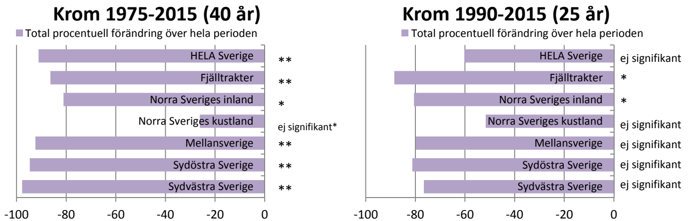
Figur 30. Trendanalys för krom i mossa uppdelat på olika regioner över Sverige för perioderna 1975-2015 och 1990-2015. Total procentuell förändring anges för perioderna. Signifikans anges i tre olika nivåer; p < 0,05 = * ; p < 0,01 = ** ; p < 0,001 = *** .
