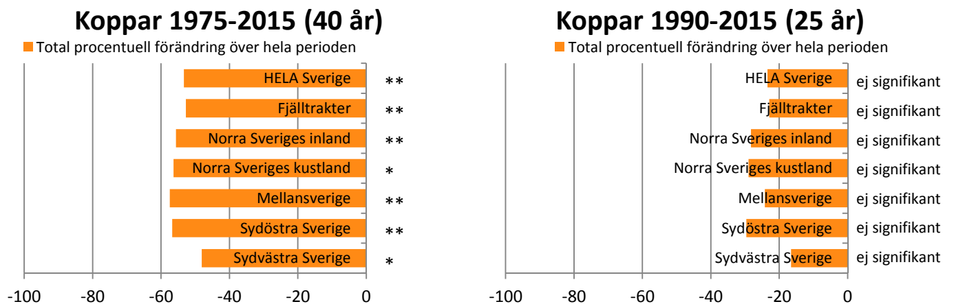
Figur 25. Trendanalys för koppar i mossa uppdelat på olika regioner över Sverige för perioderna 1975-2015 och 1990-2015. Total procentuell förändring anges för perioderna. Signifikans anges i tre olika nivåer; p < 0,05 = * ; p < 0,01 = ** ; p < 0,001 = *** .
