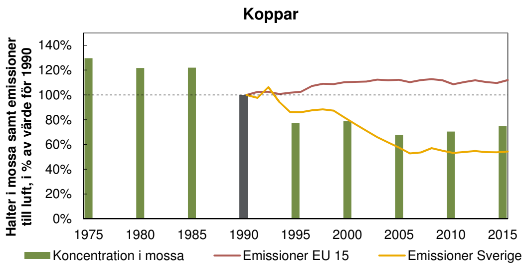
Figur 24. Medelkoncentration av koppar i mossa sedan 1975 för Sverige samt emissioner av koppar till luft för Sverige och Europa (EU15) sedan 1990. Koncentration i mossa visas som procent av 1990 års värde.
