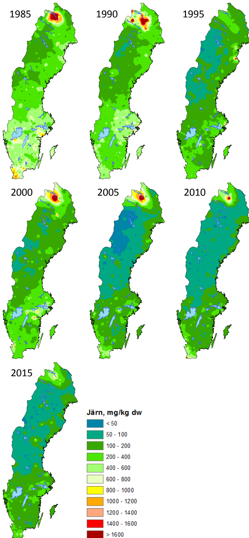
Figur 14. Koncentration (mg/kg torrsvikt) av järn i mossor, 1985-2015.
