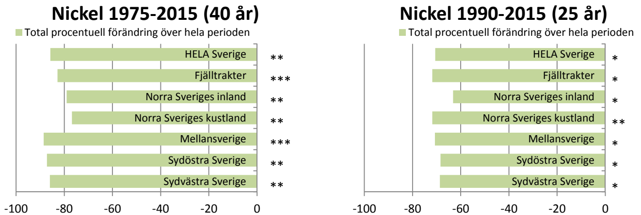
Figur 39. Trendanalys för nickel i mossa uppdelat på olika regioner över Sverige för perioderna 1975-2015 samt 1990-2015. Total procentuell förändring anges för perioderna. Signifikans anges i tre olika nivåer; p < 0,05 = * ; p < 0,01 = ** ; p < 0,001 = *** .
