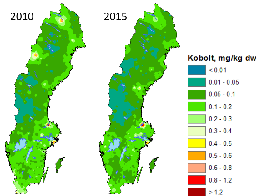
Figur 54. Koncentration (mg/kg torrsvikt) av kobolt i mossor, 2010 och 2015.
