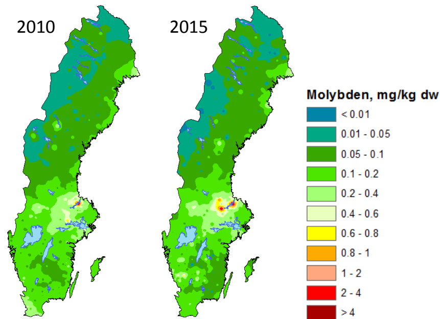
Figur 60. Koncentration (mg/kg torrsvikt) av molybden i mossor, 2010 och 2015.
