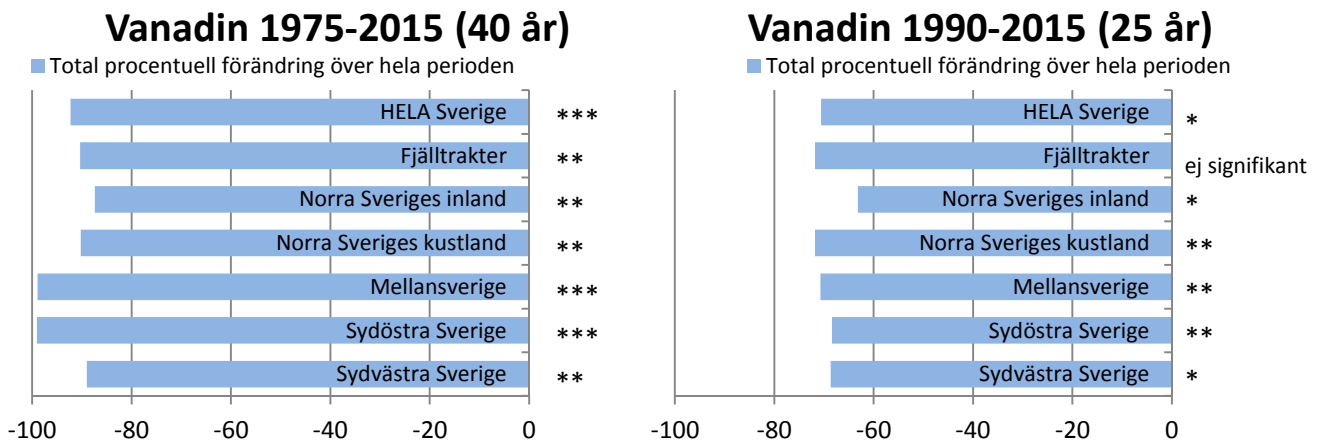
Figur 43. Trendanalys för vanadin i mossor uppdelat på olika regioner över Sverige för perioderna 1975-2015 och 1990-2015. Total procentuell förändring anges för perioderna. Signifikans anges i tre olika nivåer; p < 0,05 = * ; p < 0,01 = ** ; p < 0,001 = *** .
