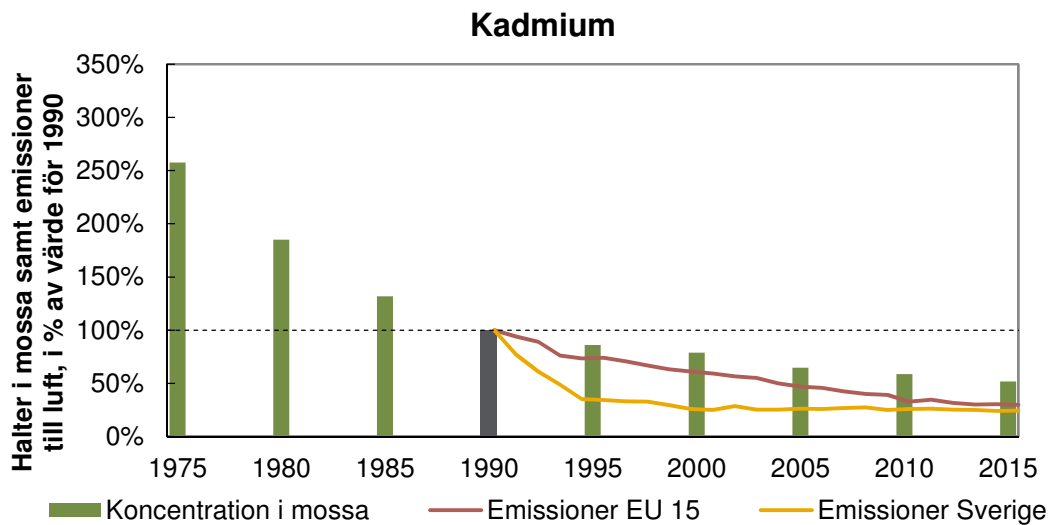
Figur 19 Medelkoncentration av kadmium i mossa sedan 1975 för Sverige samt emissioner av kadmium till luft för Sverige och Europa (EU15) sedan 1990. Koncentration i mossa och emissioner till luft visas som procent av 1990 års värde.
