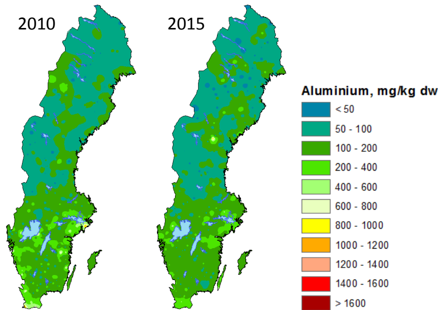
Figur 51. Koncentration (mg/kg torrsvikt) av aluminium i mossor, 2010 och 2015.
