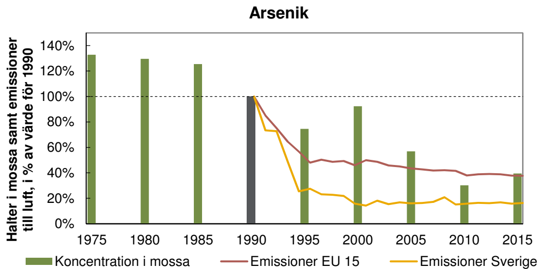
Figur 5. Medelkoncentration av arsenik i mossor sedan 1975 för Sverige samt emissioner av arsenik till luft för Sverige och Europa (EU15) sedan 1990. Koncentration i mossor och emissioner till luft visas som procent av 1990 års värde.
