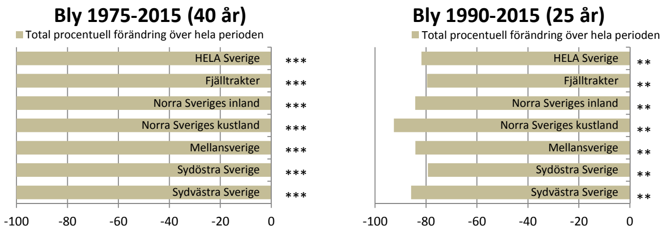
Figur 11. Trendanalys för bly i mossa uppdelat på olika regioner över Sverige för perioderna 1975-2015 och 1990-2015. Total procentuell förändring anges för perioderna. Signifikans anges i tre olika nivåer; p < 0,05 = * ; p < 0,01 = ** ; p < 0,001 = *** .
